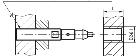
Схема монтажа
